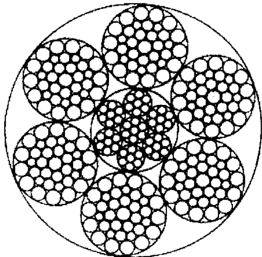
6×36WS+IWR
