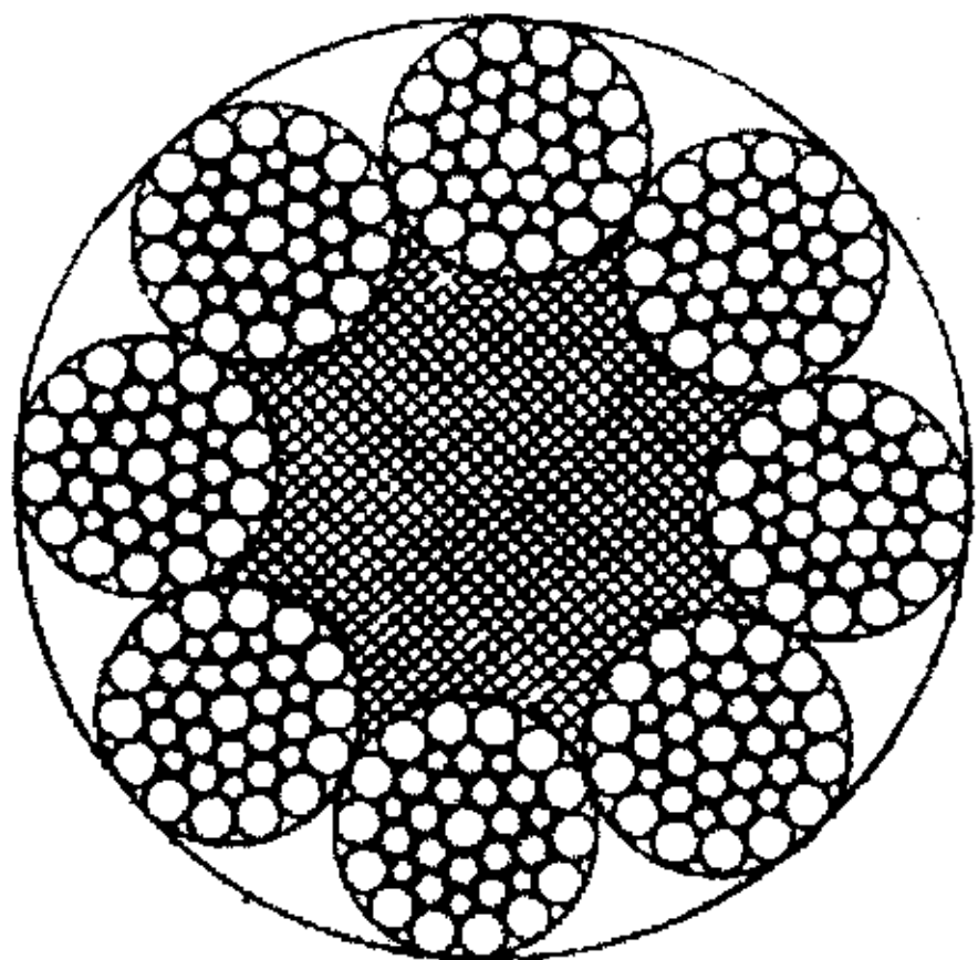
8×36WS+FC
