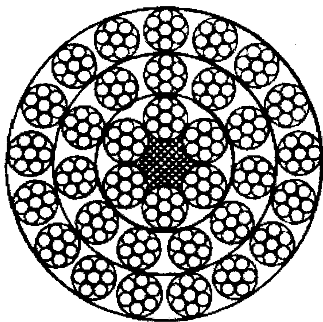
34×7+FC
