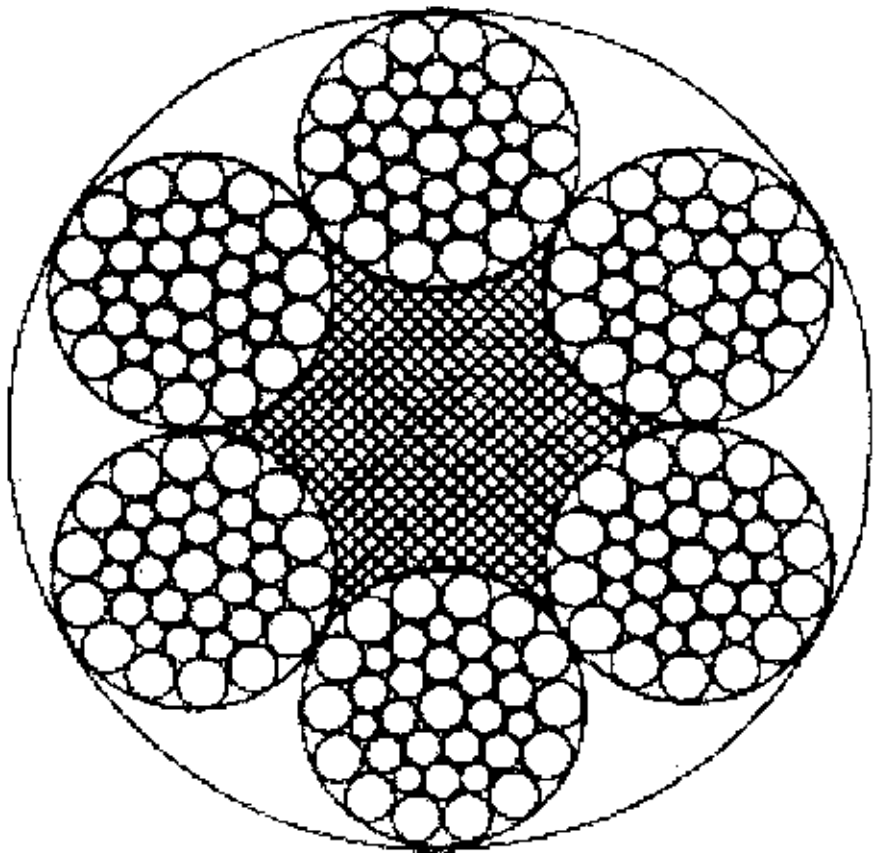
6×36WS+FC
