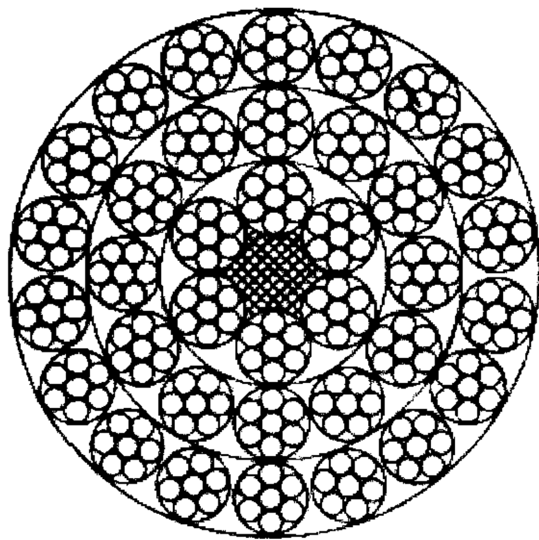
36×7+FC
