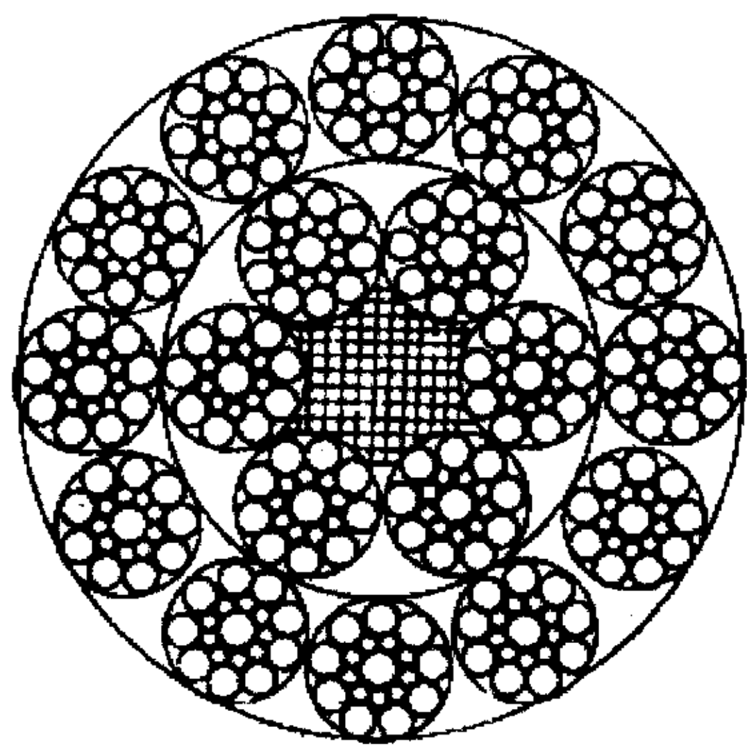
18×19S+FC
