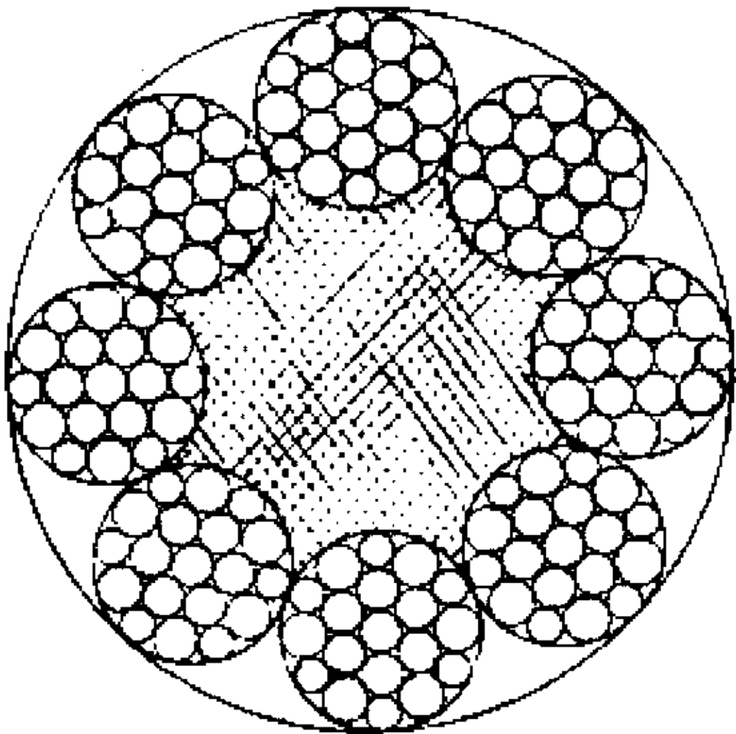
8×19W+FC
