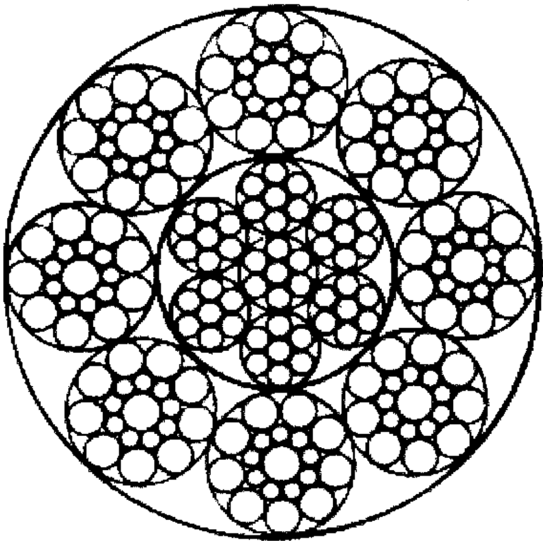
8×19S+IWR
