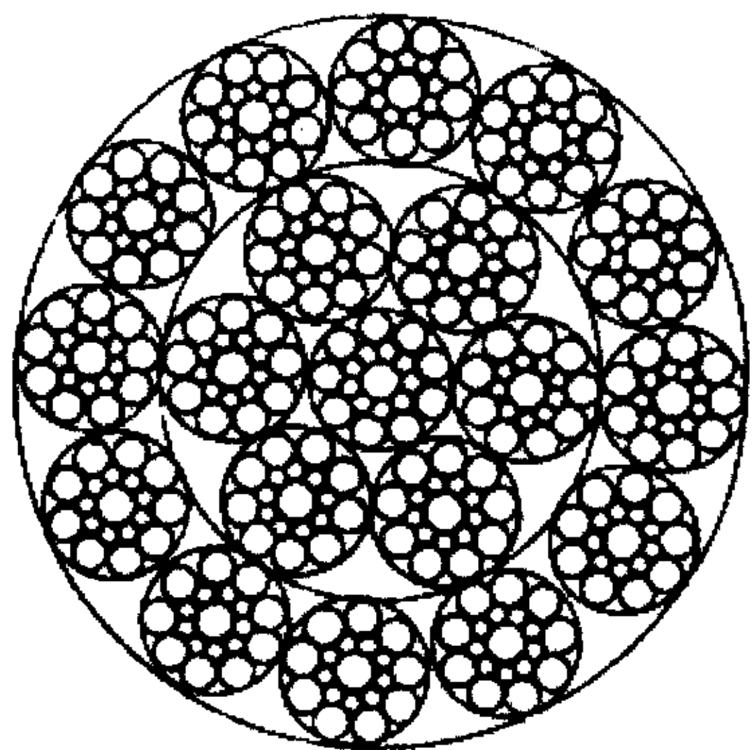
18×19S+IWS
