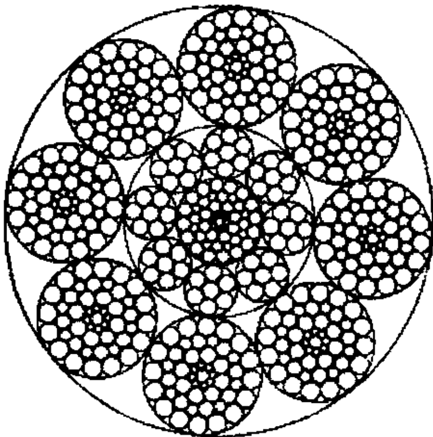
8×49SWS+IWR
