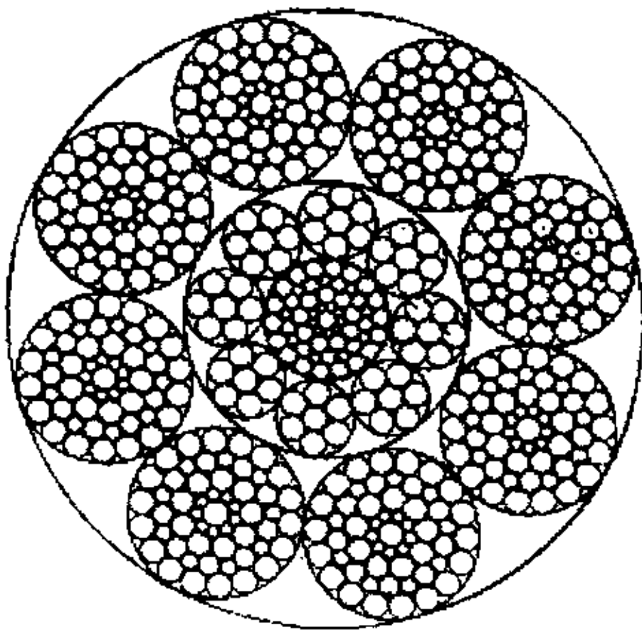
8×55SWS+IWR
