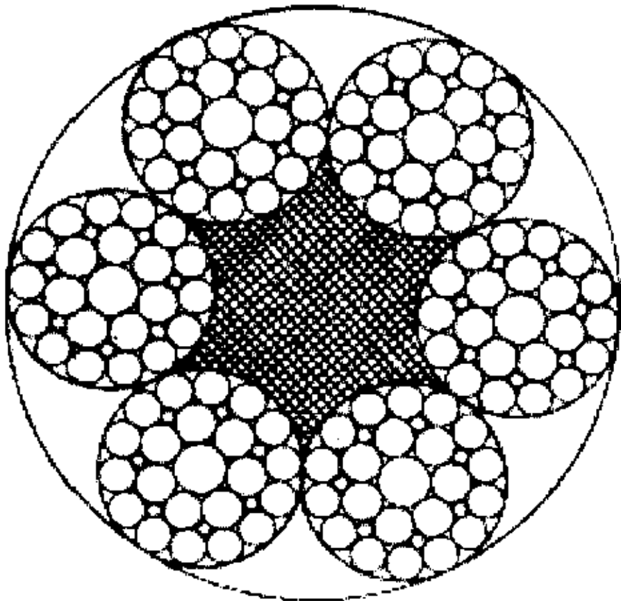
6×29Fi+FC
