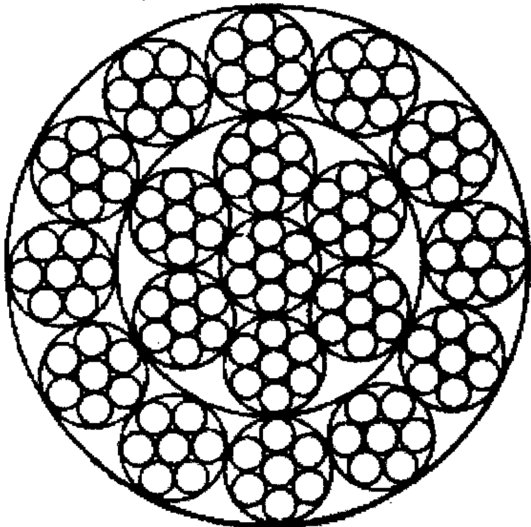
18×7+IWS
