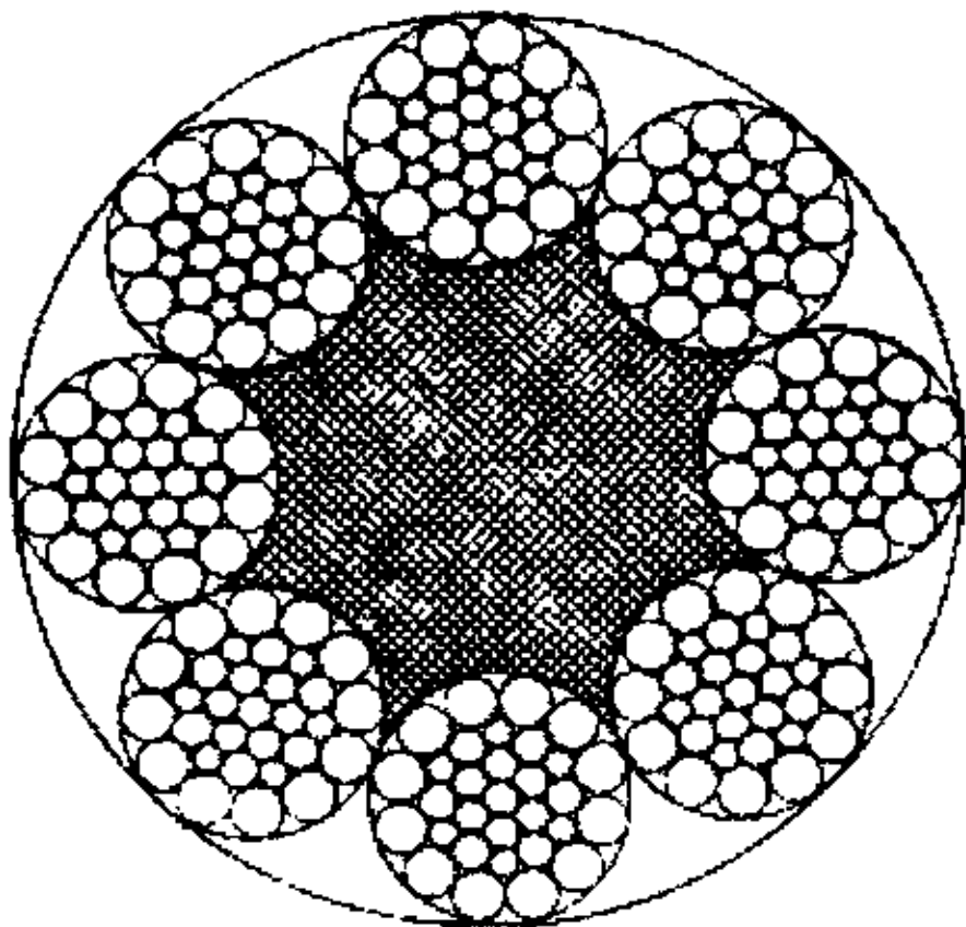
8×31WS+FC
