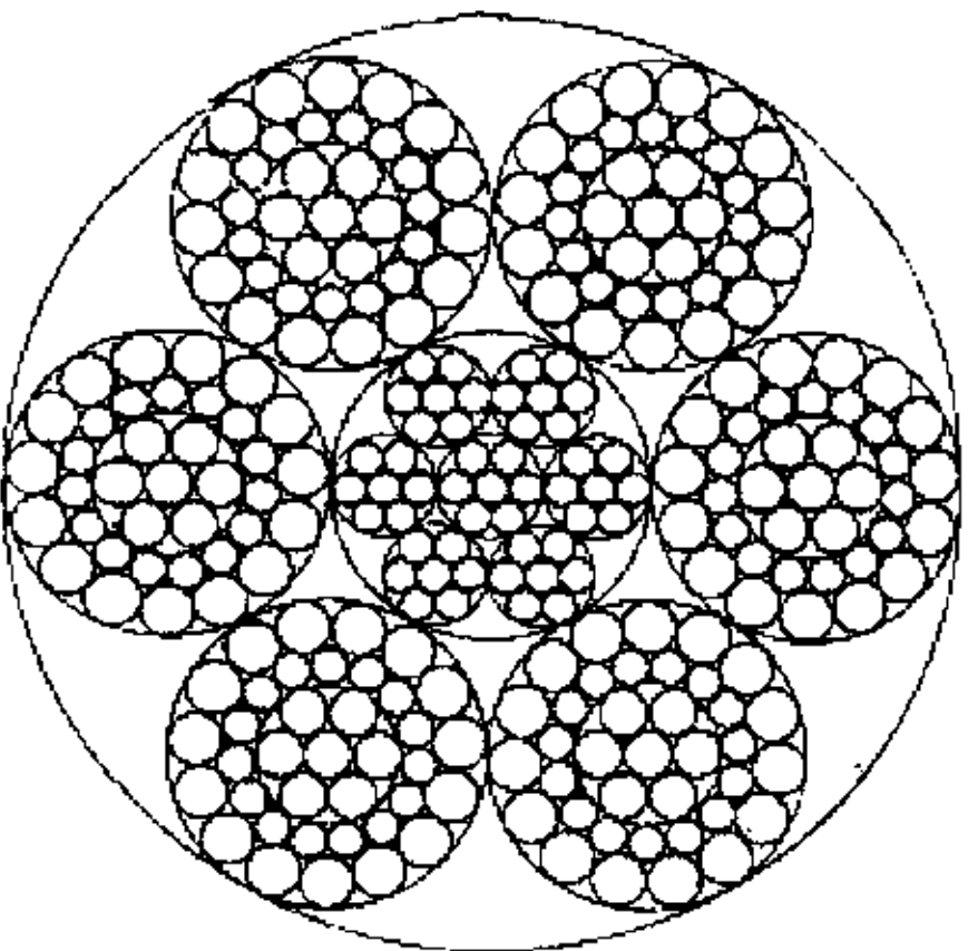
6×37S+IWR
