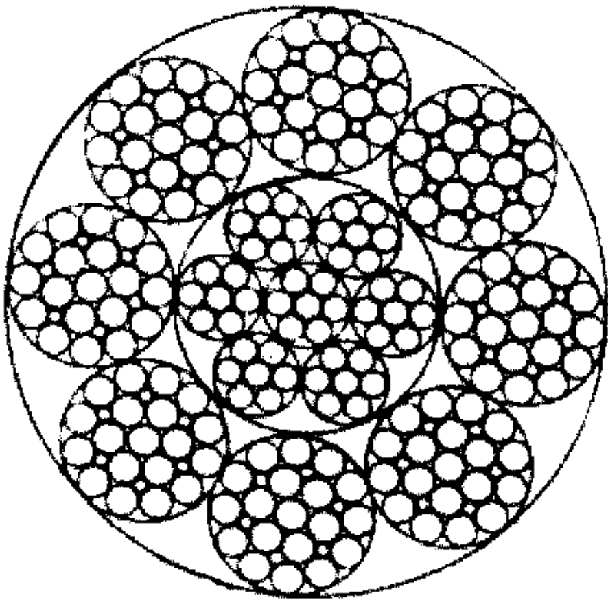
8×25Fi+IWR
