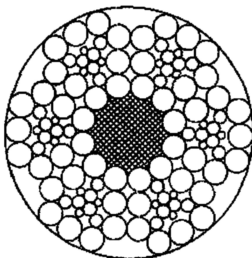
6V×18+FC
