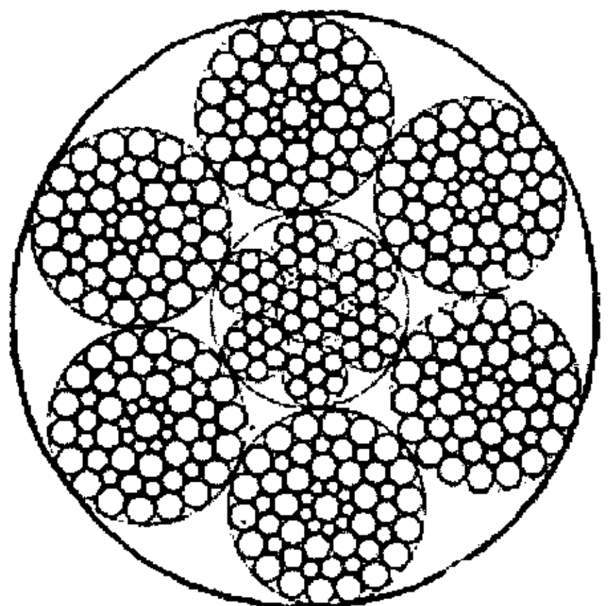
6×55SWS+IWR
