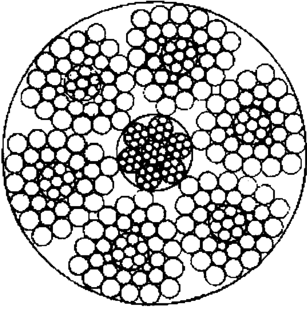
6V×37S+IWR
