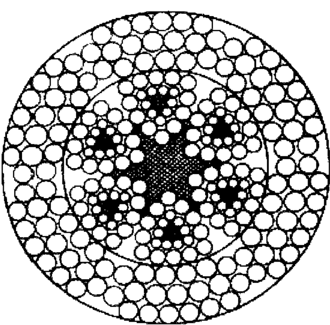
6Q×19+6V×21+7FC 直径:40 mm~52 mm
