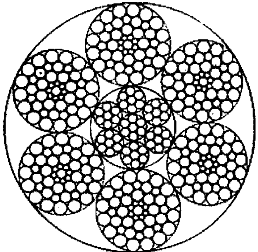
6×49SWS+IWR
