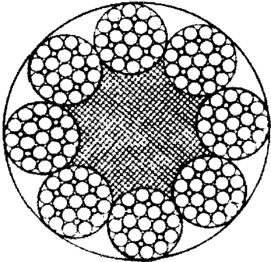
8×25Fi+FC
