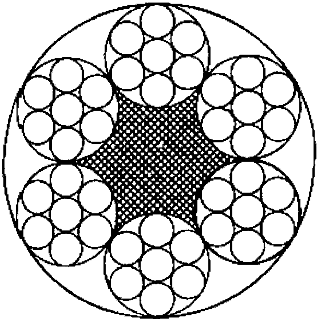
6×7+FC
