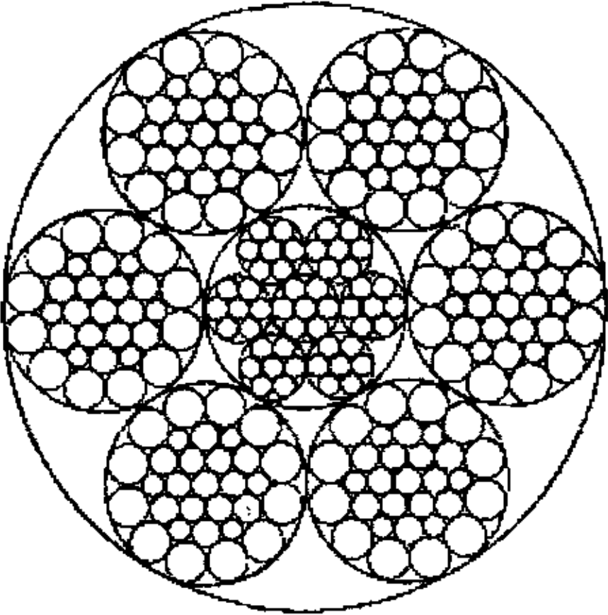
6×31WS+IWR
