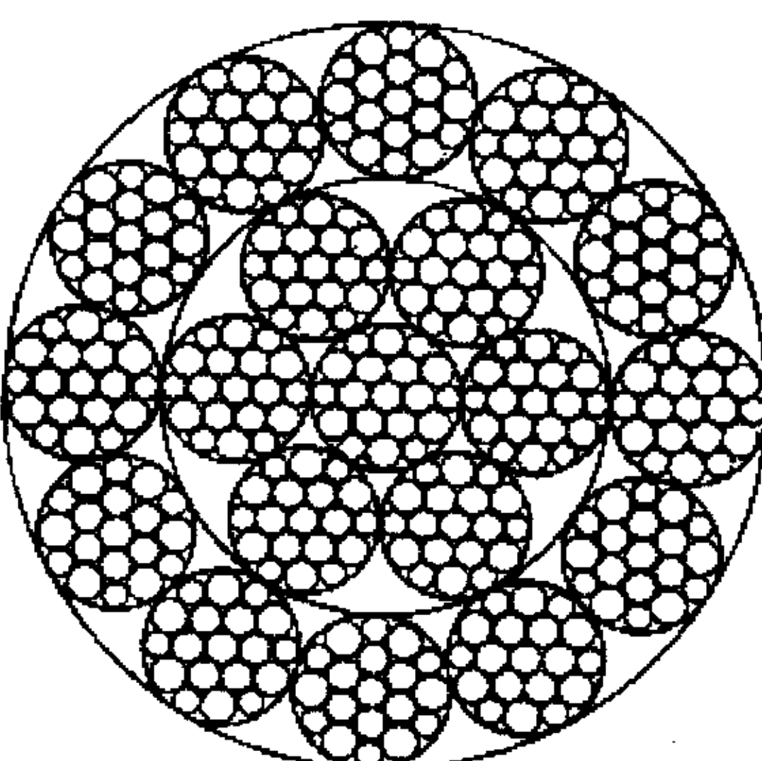
18×19W+IWS
