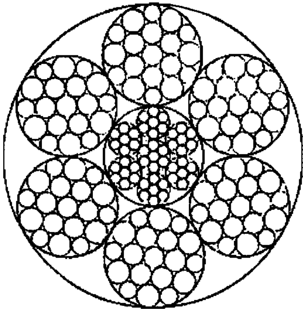
6×19W+IWR
