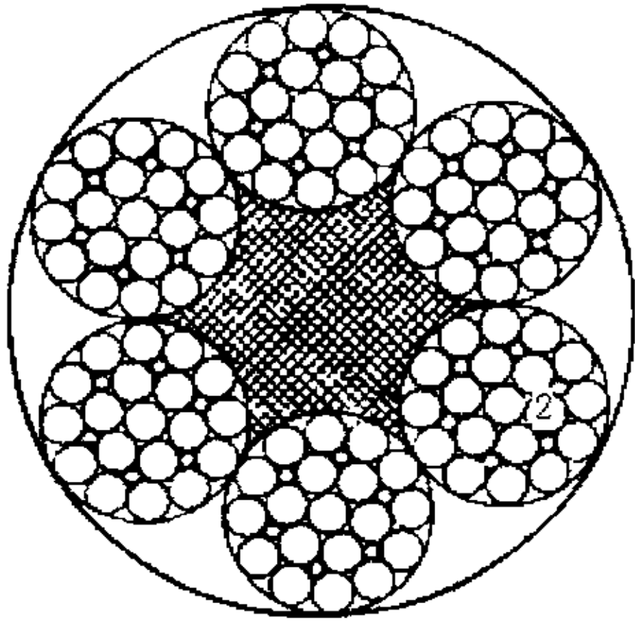
6×25Fi+FC
