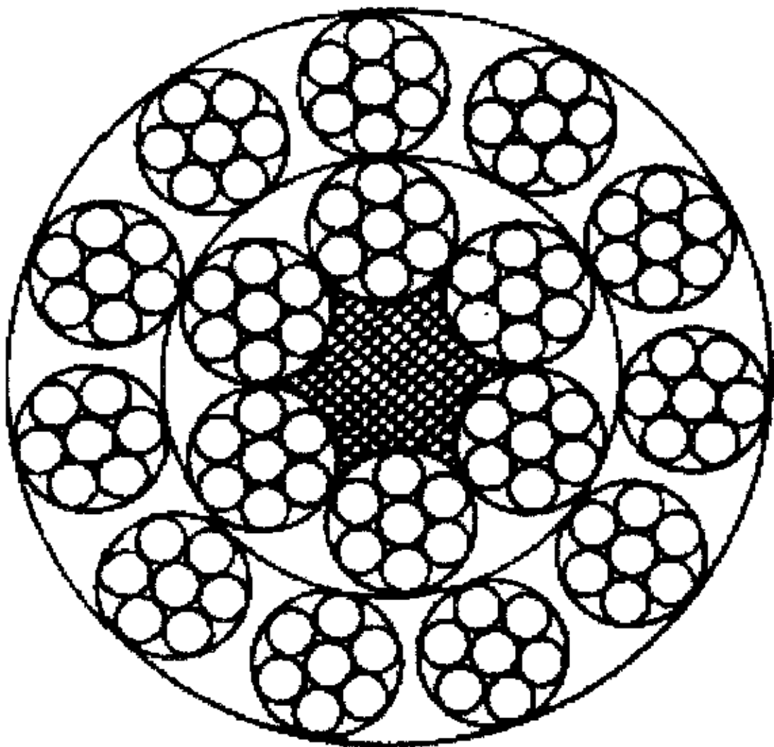
17×7+FC
