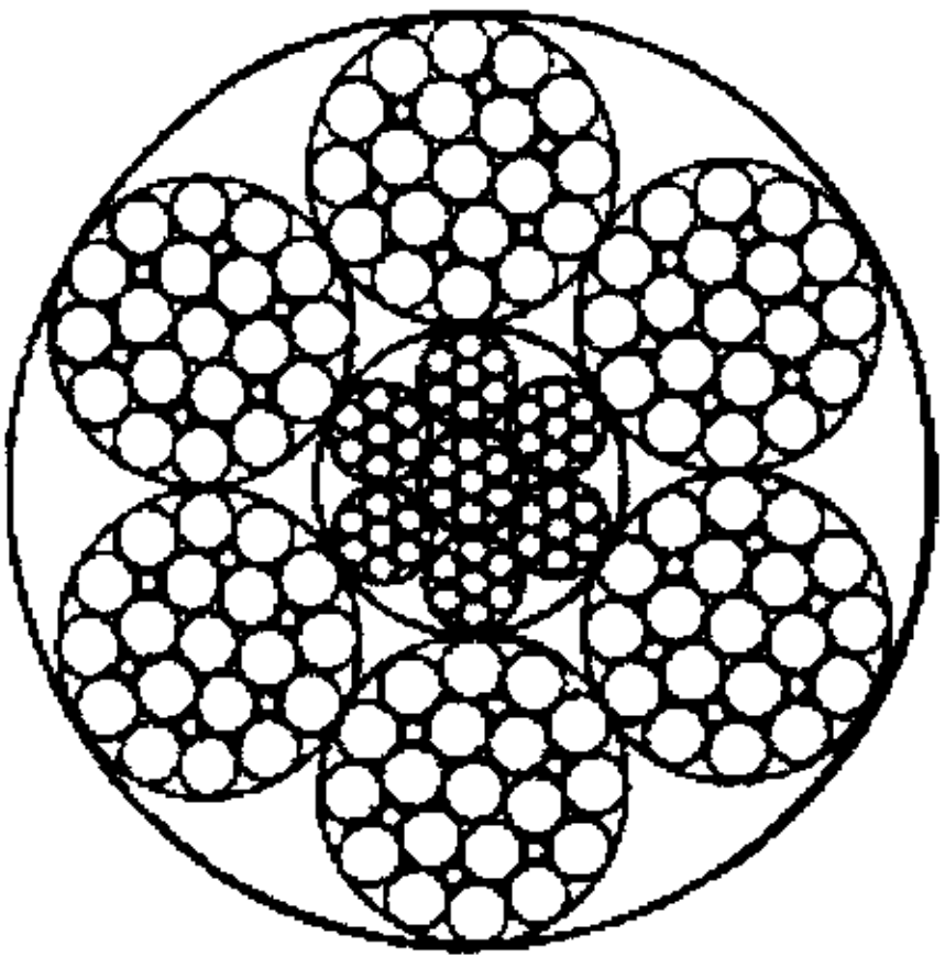
6×25Fi+IWR
