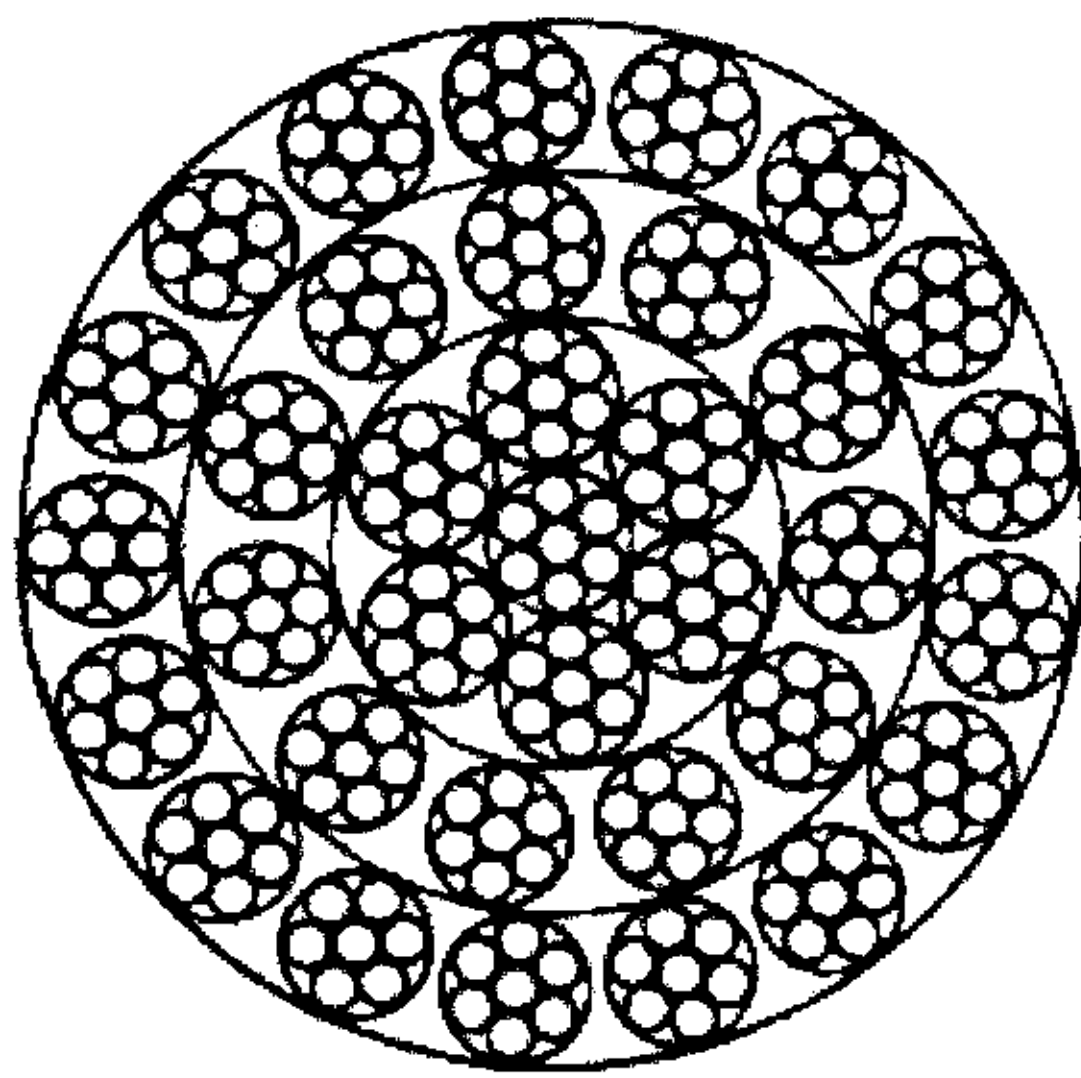
34×7+IWS
