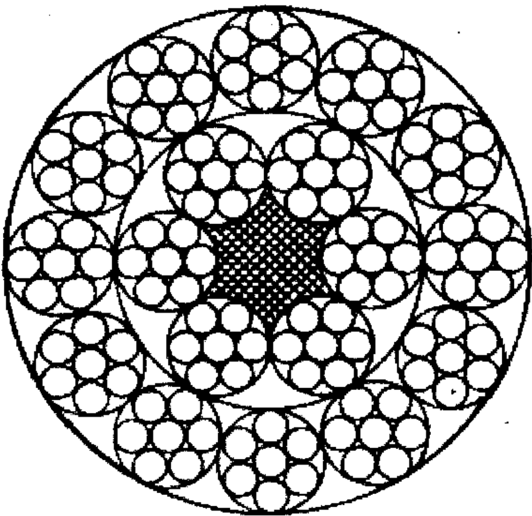
18×7+FC
