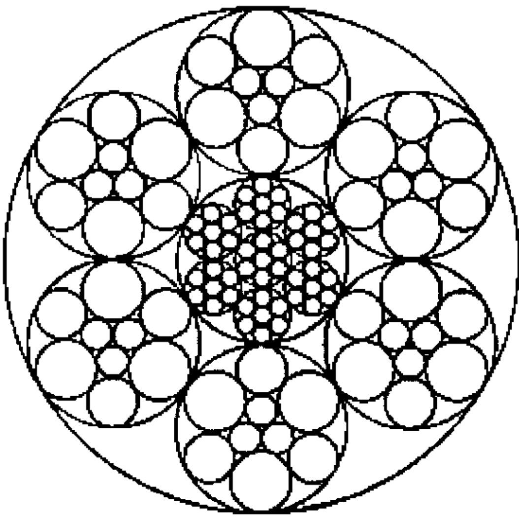
6×9W+IWR
