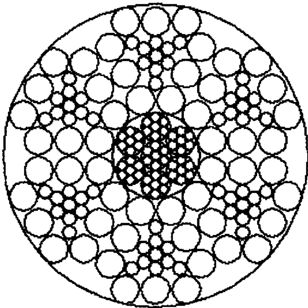
6V×19+IWR
