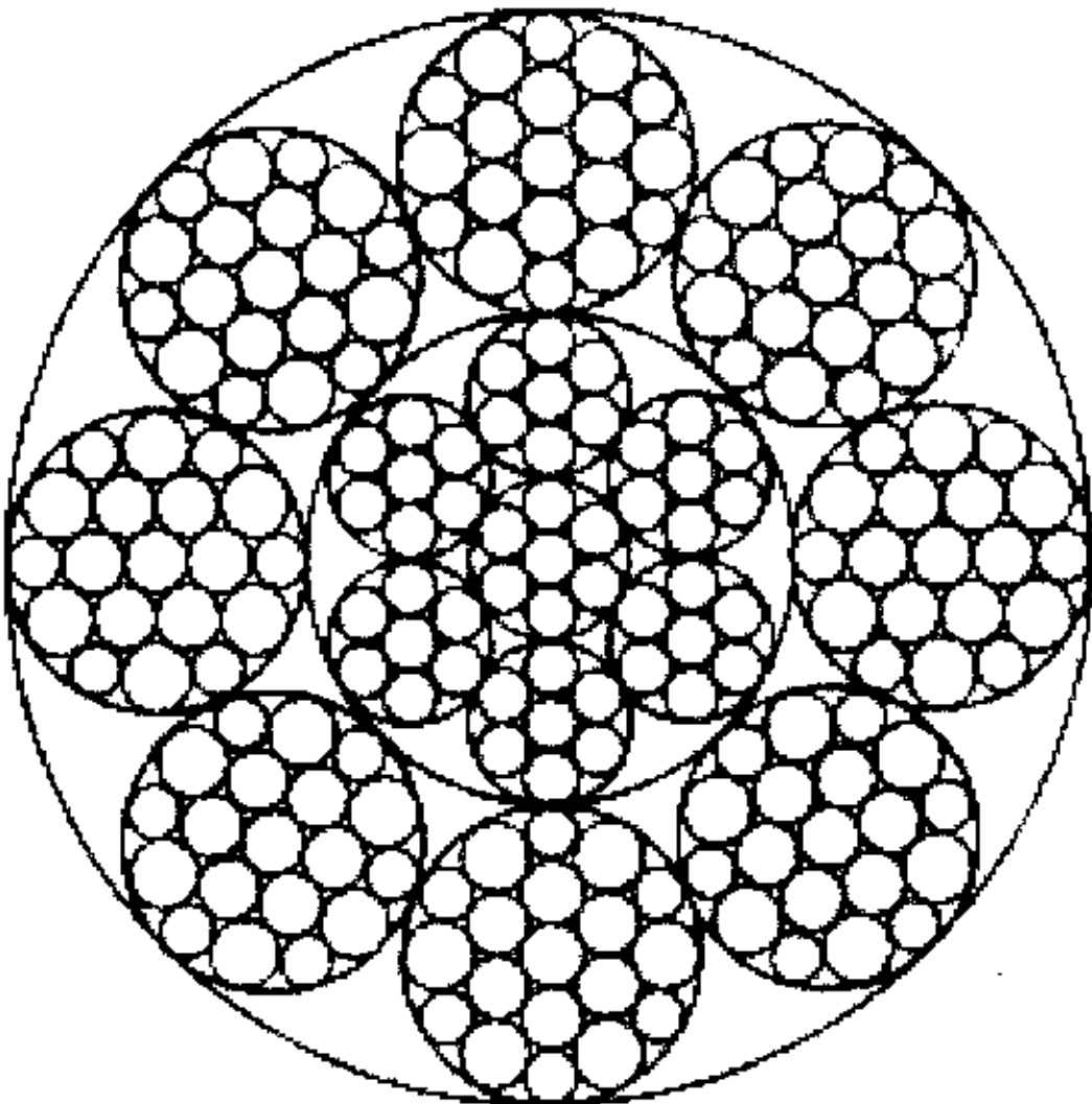
8×19W+IWR
