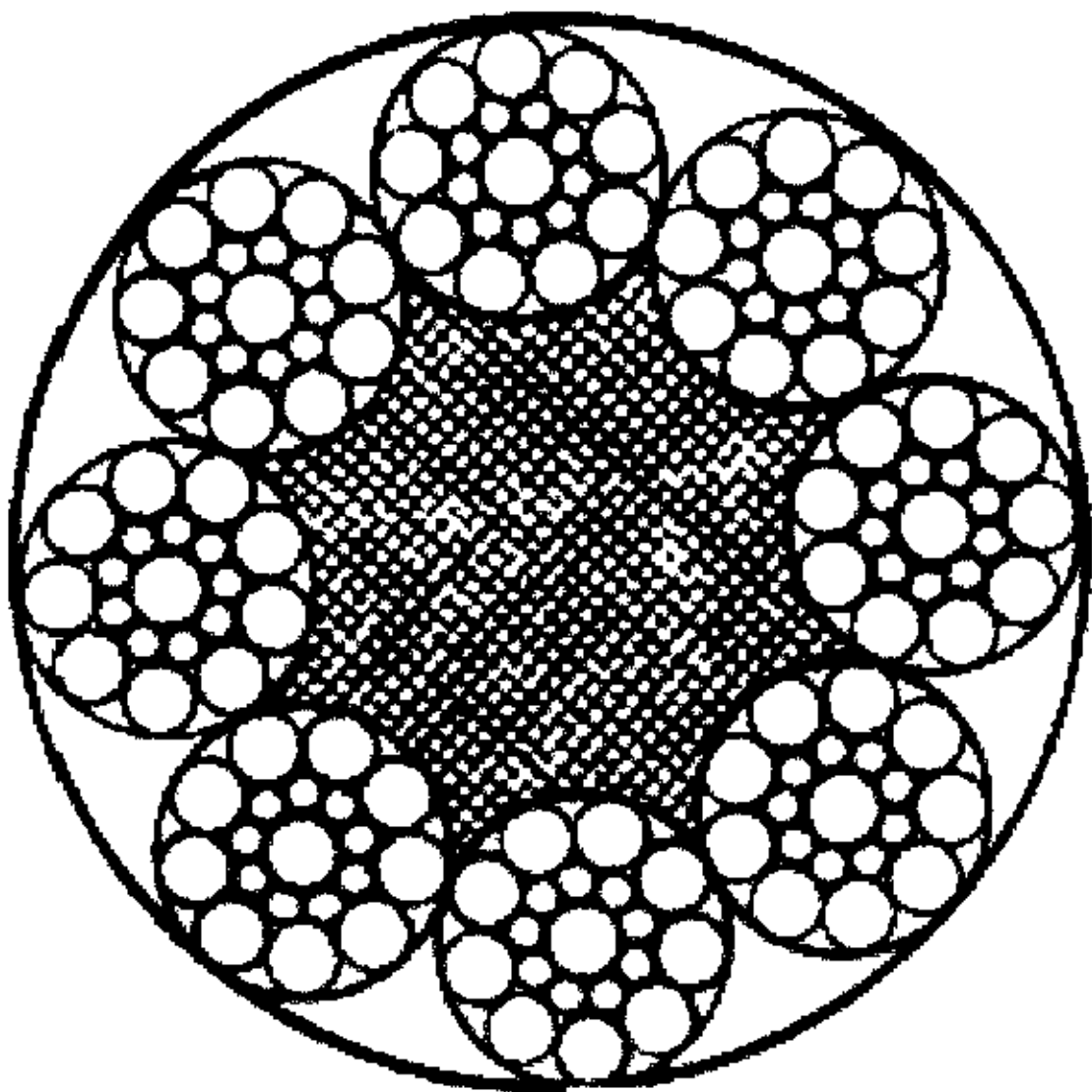
8×19S+FC
