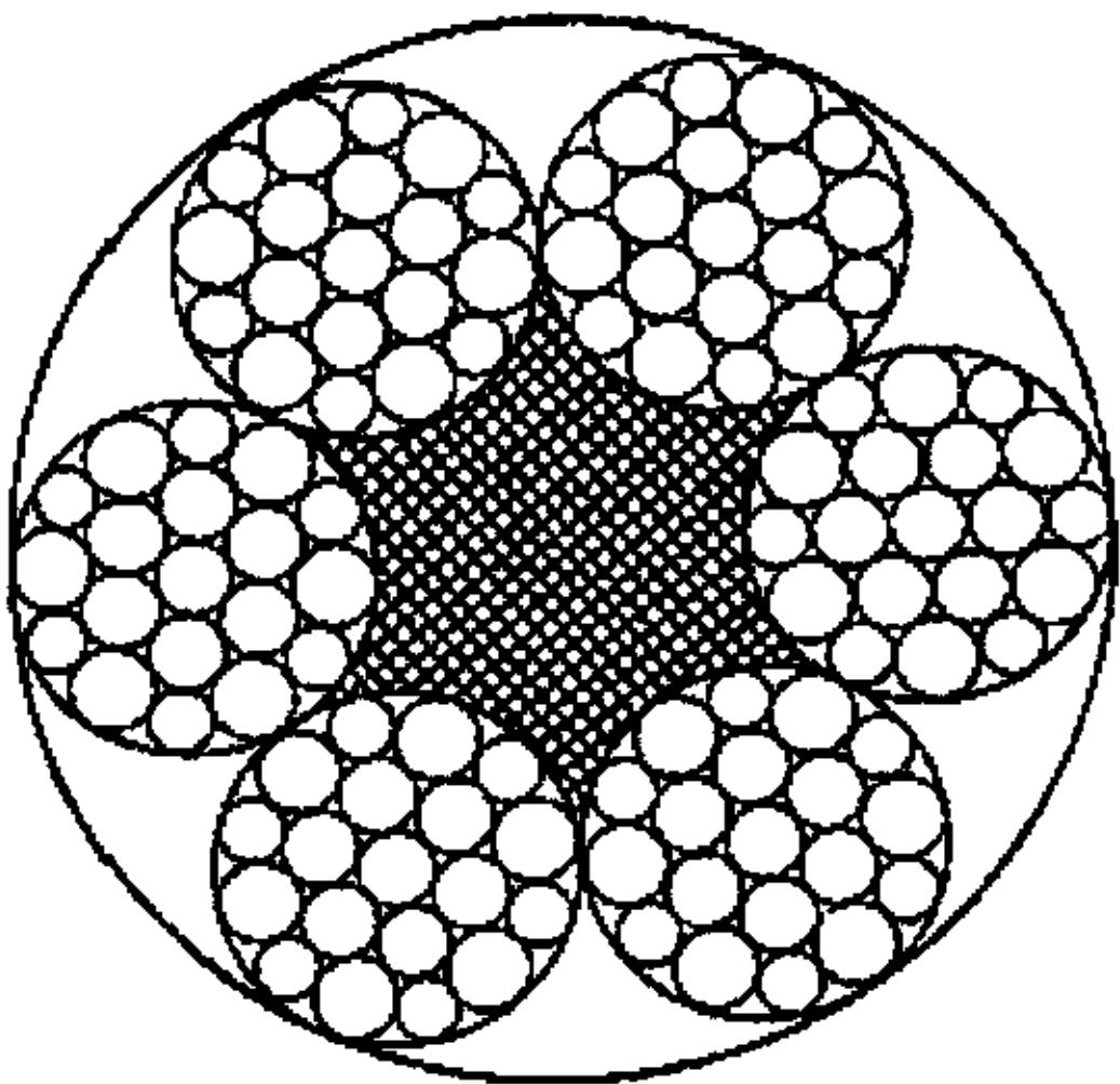
6×19W+FC
