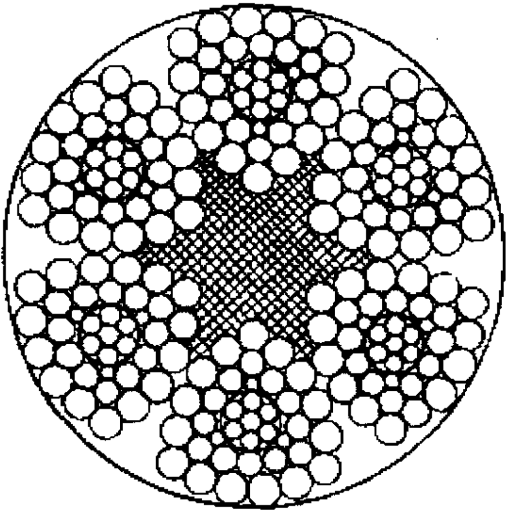
6V×37S+FC
