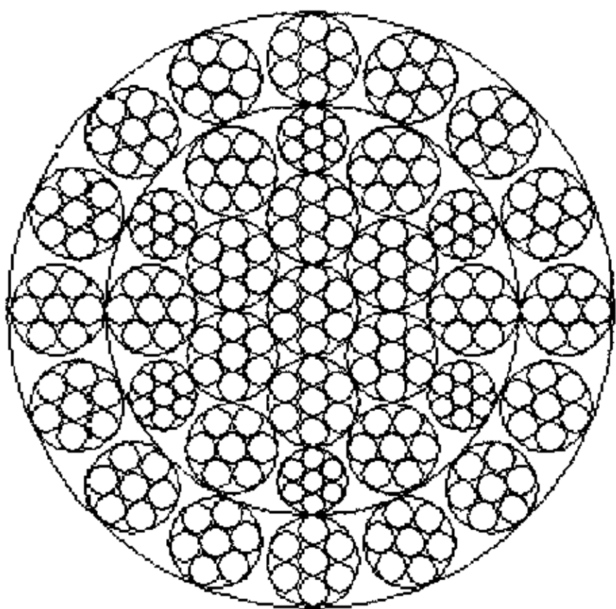
35W×7
