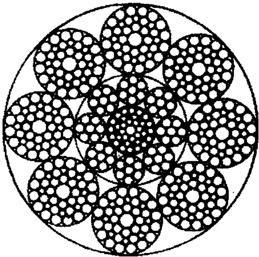
8×41WS+IWR
