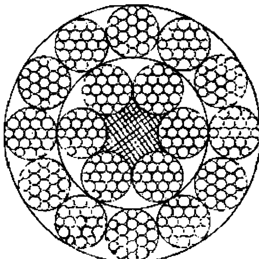
18×19W+FC
