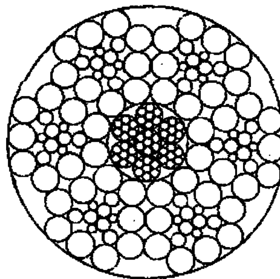
6V×18+IWR
