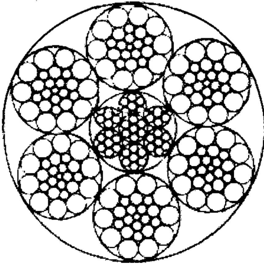
6×26WS+IWR
