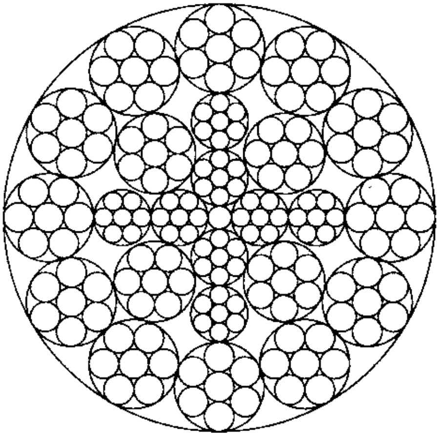
24W×7
