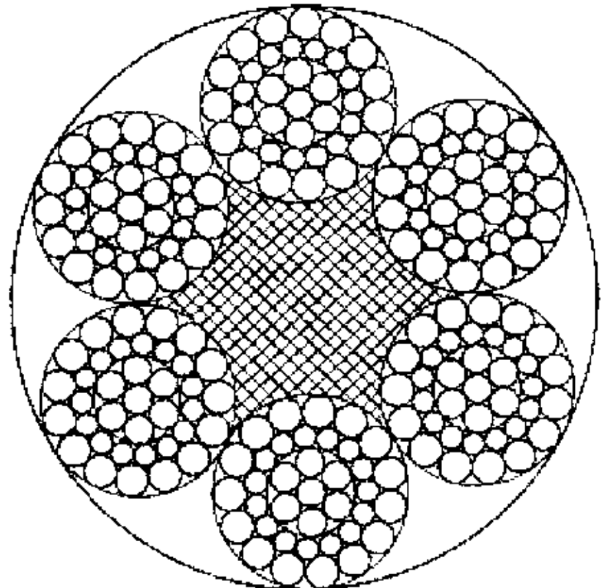
6×37S+FC
