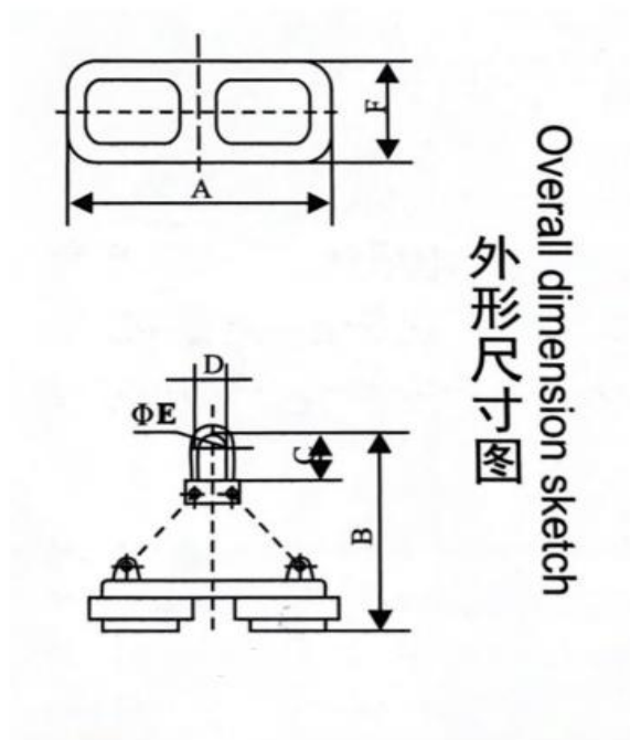
MW16 (MW96) 系列（额定电压DC-220V，通电持续率TD-50%）主要技术参数 Main technical parameters of MW16 (MW96) series (rated voltage DC-220V, TD-50%)
